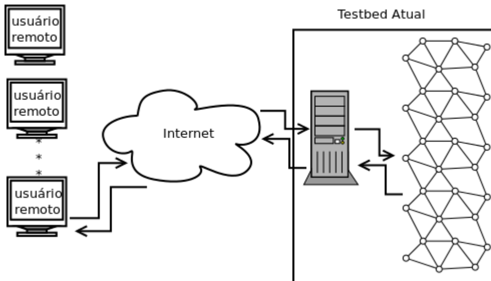
Figura 3: Arquitetura geral do piloto.
