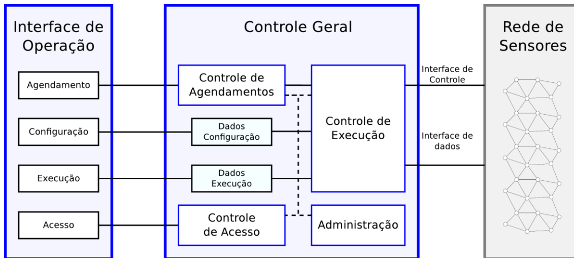
Figura 2: Arquitetura funcional do testbed.
