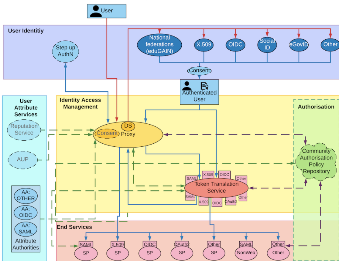
Figura 1. Modelo de Arquitetura AARC
