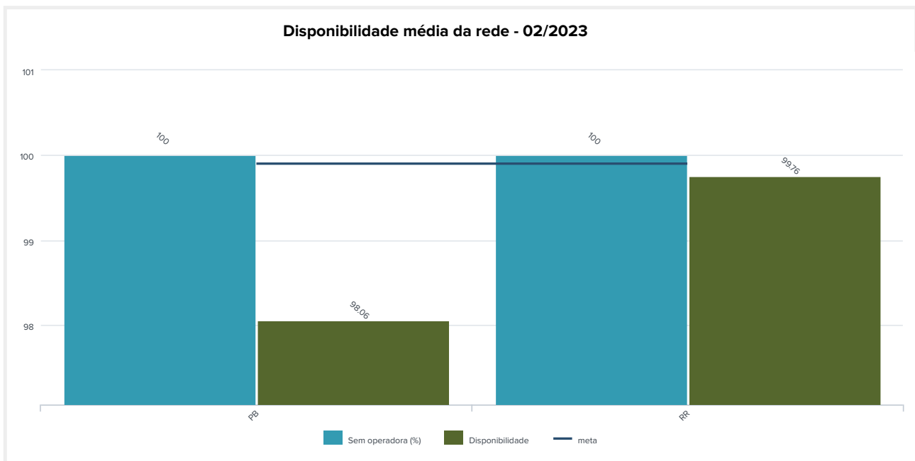
Figura 12: Disponibilidade para alguns PoPs, com e sem contribuição de suas operadoras, em fevereiro de 2023.
