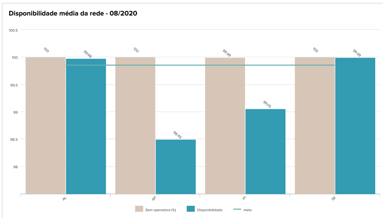
Figura 12: Disponibilidade para alguns PoPs, com e sem contribuição de suas operadoras, em agosto de 2020.
